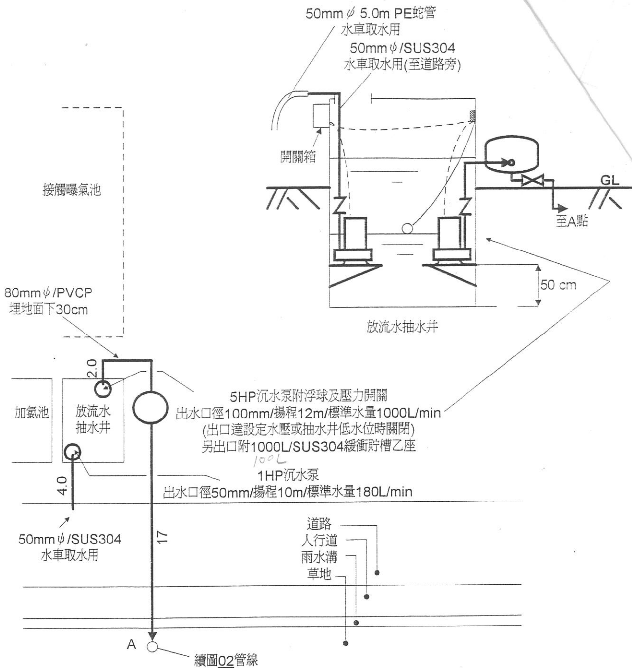
圖 01: 設備配置圖.
