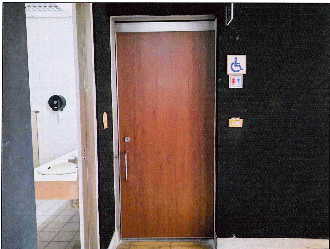
照片(8)、文學院藝術大樓 2F 東側無障礙兼性別友善廁所無障礙廁所橫拉門(含五金配件)
